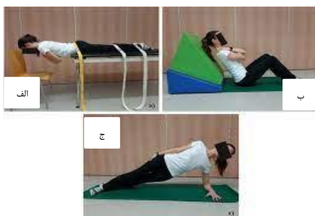
شکل ۱. الف) آزمون سورنس؛ ب) آزمون V؛ ج) آزمون پلانک
